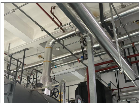
锅炉房可燃气体报警器
