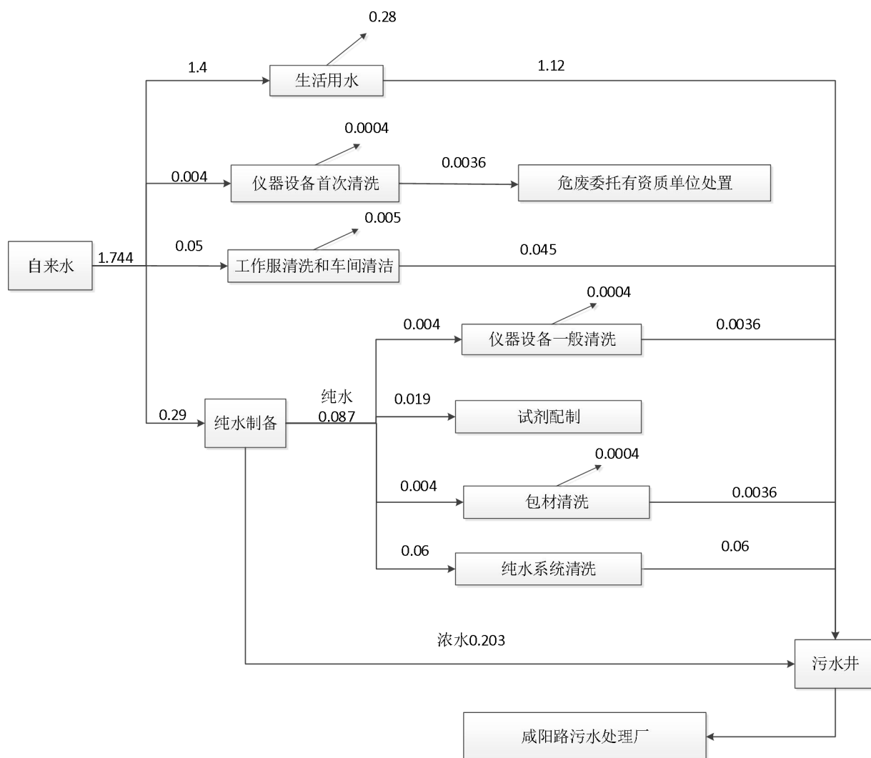
图 1-2 项目水平衡图 m³/d
