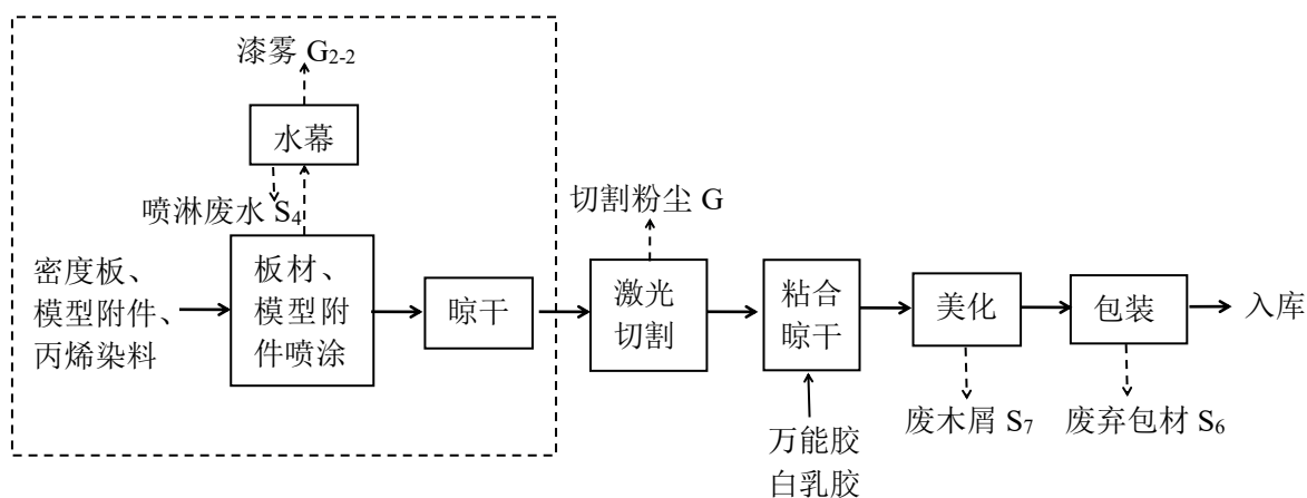
图 3.6-2 工艺品模型生产工艺流程图
