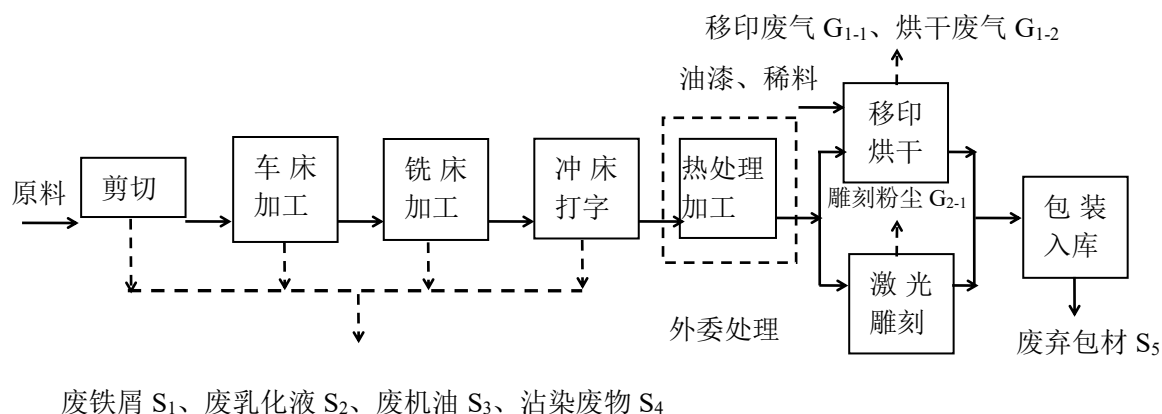
图 3.6-1 批咀、套筒生产工艺流程图
