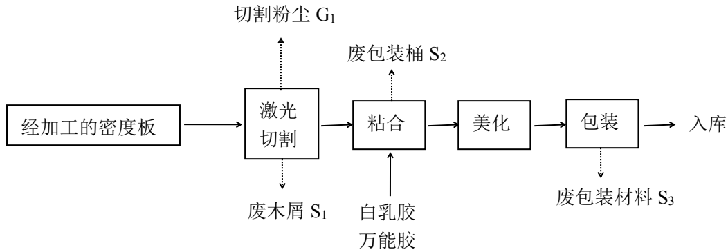
图 3.5-1 工艺品模型工艺流程图
